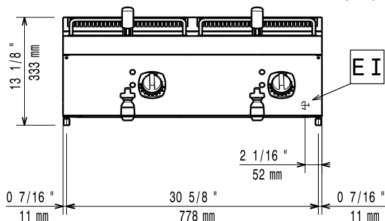
Előlnézet
