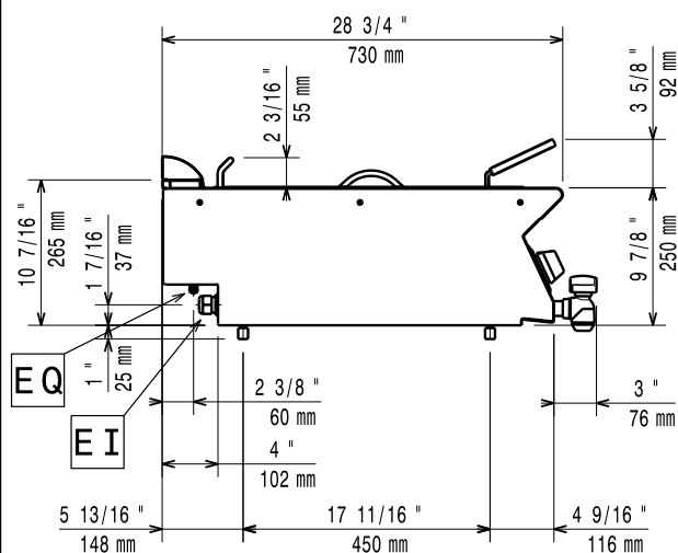
Oldalnézet
